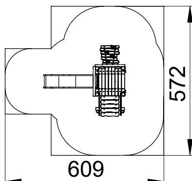
plattegrond
